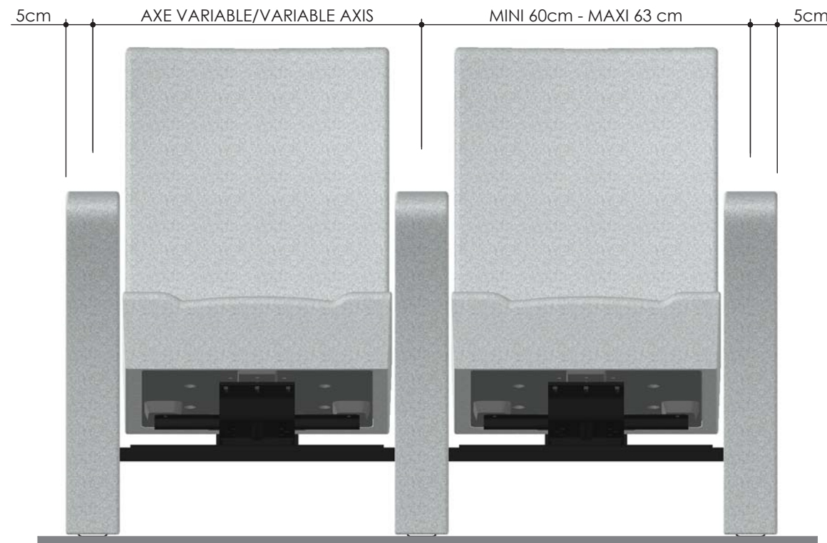
VUE DE FACE - FRONT VIEW
