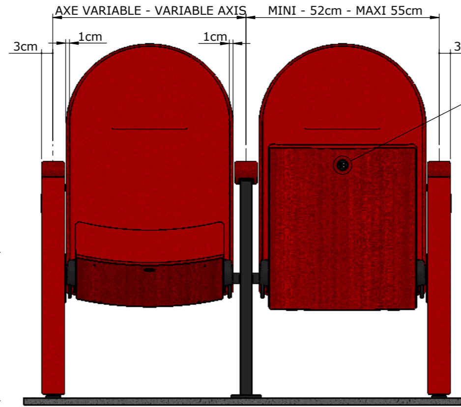
VUE DE FACE / FRONT VIEW
