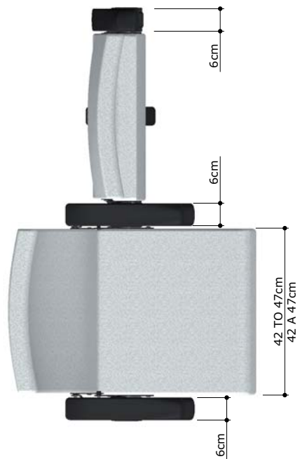
VUE DE DESSUS / TOP VIEW
